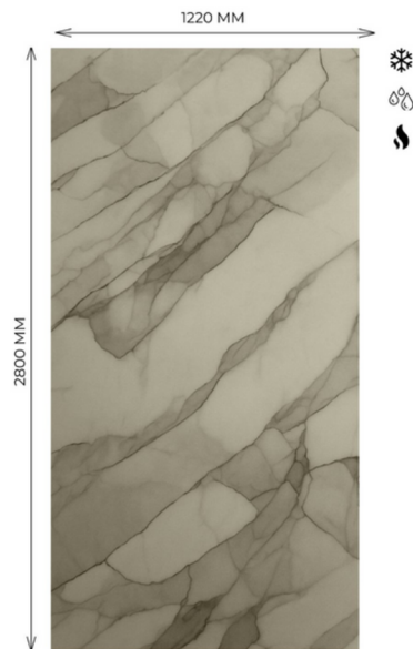
Панель ПВХ №61Ts-115 (2800x1220x3), вес 19 кг
